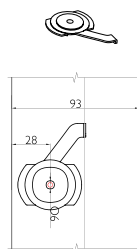
sdužené rolety
