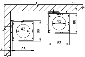
zátěžová lišta
